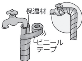
＜図1＞ むき出しの水道管の防寒方法
