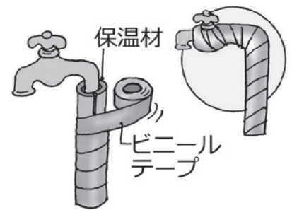
＜図1＞むき出しの水道管の防寒方法
