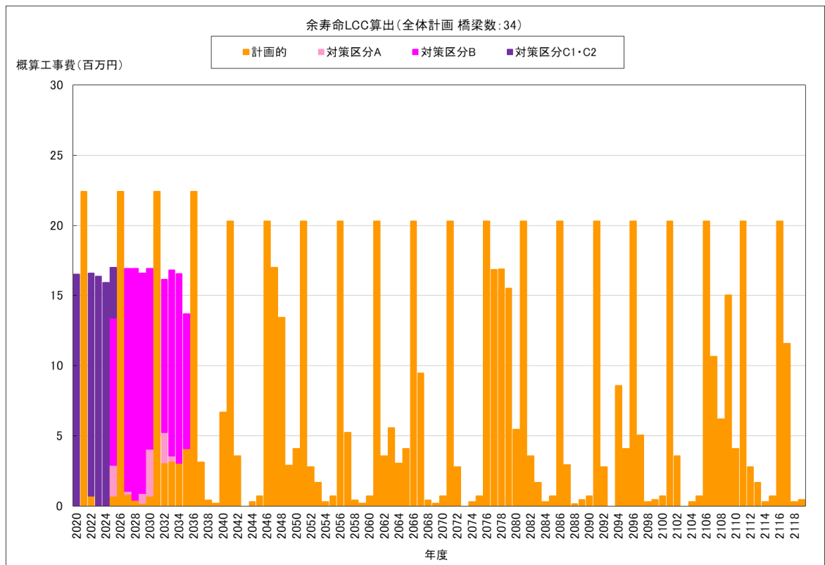
図 7-3 予算平準化による算出結果
