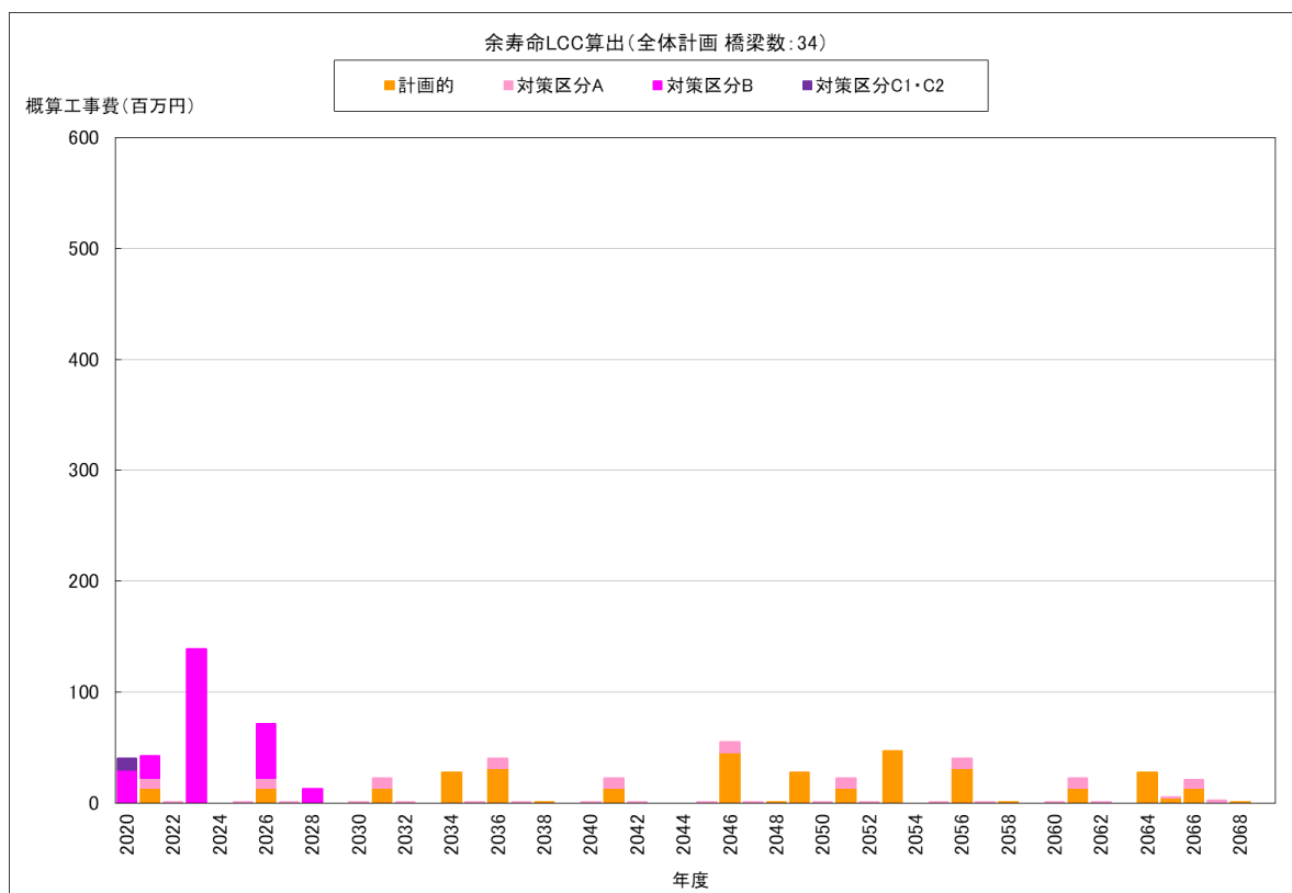
図 7-1 予防保全型の LCC 算出結果
